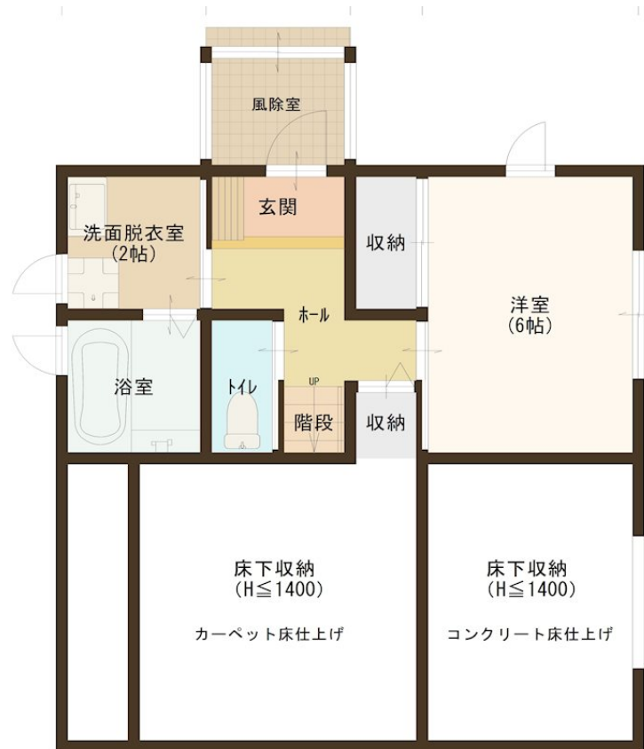
【間取り図】
