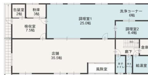
【間取り図】
