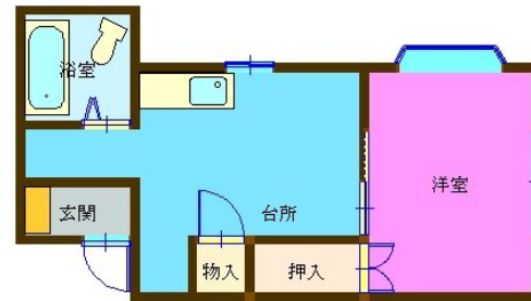
【間取り図】
