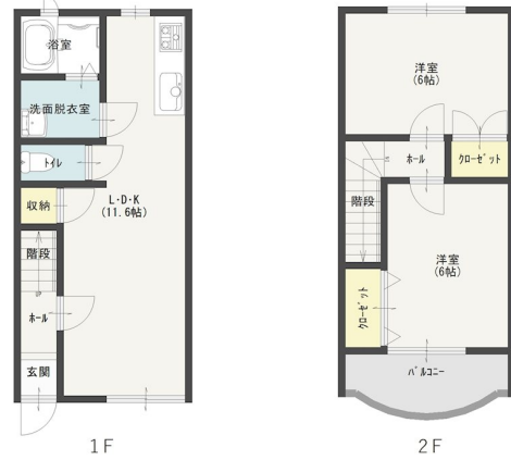
【間取り図】
