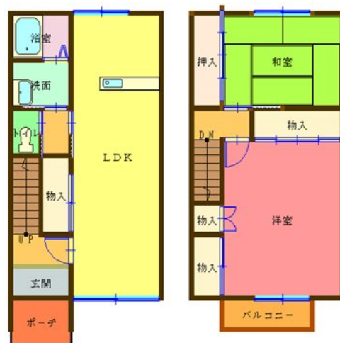
【間取り図】
