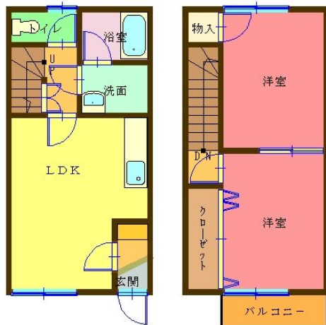
【間取り図】
