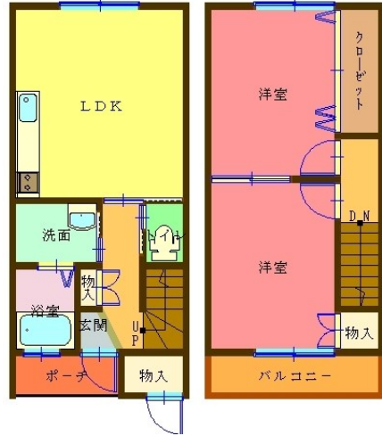
【間取り図】
